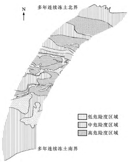
图 6 青藏高原多年冻土区危险度识别结果
