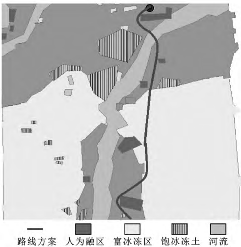
图 12 路线设计结果
