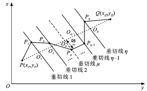
图 7 公路平面线形模型
